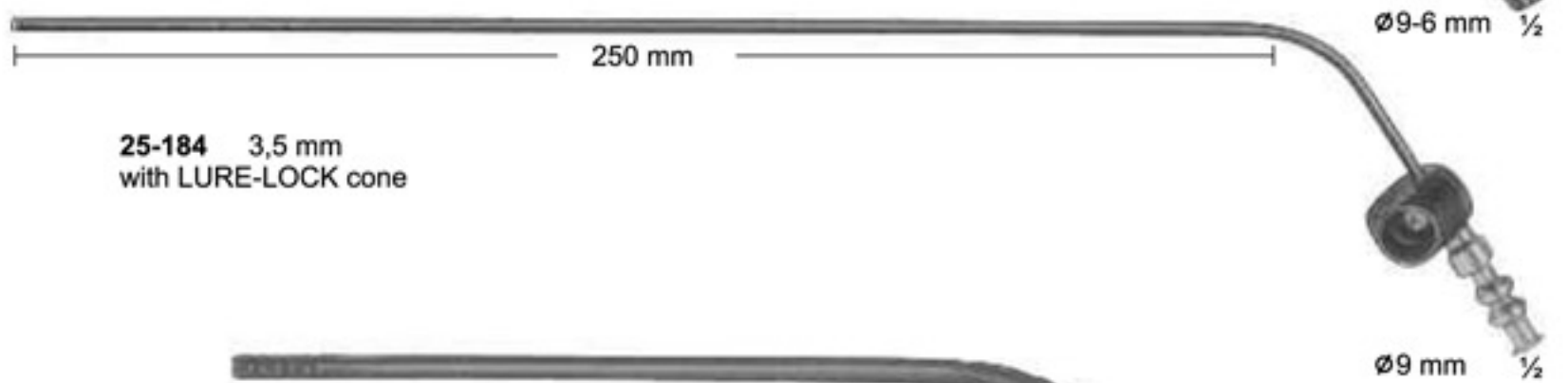
25-181 - 183 HOUSE suction tube diam. irrigation tube Diam. 25-181 0,9 mm 0,7 mm 25-182 1,2 mm 0,9 mm 25-183 1,5 mm 1,2 mm with finger cut-off and stylet, with LURE hub
